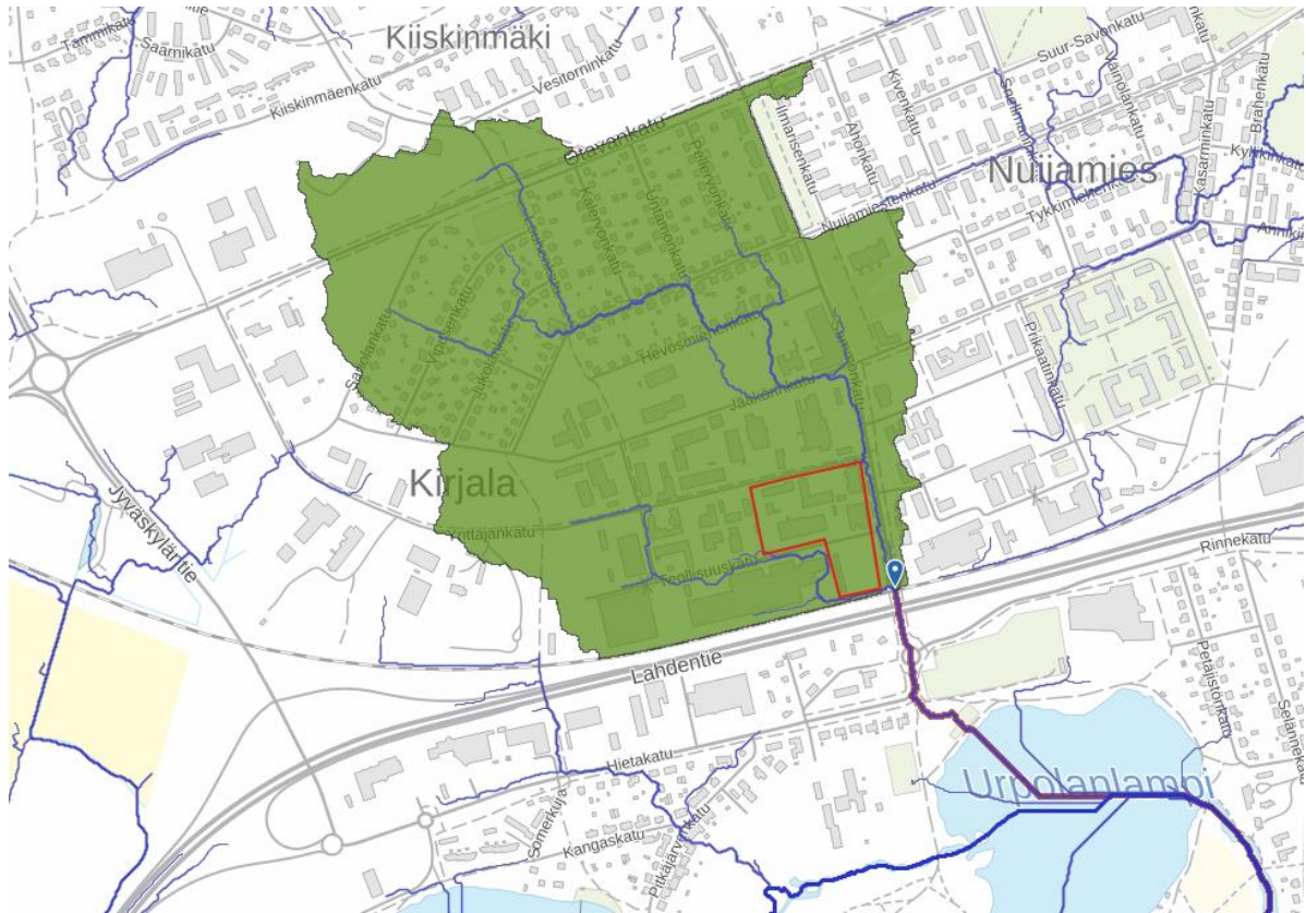
Kuva 5. Valuntareitit suunnittelualueella sinisellä (SCALGO 2024). Suunnittelualan rajausta punaisella.
