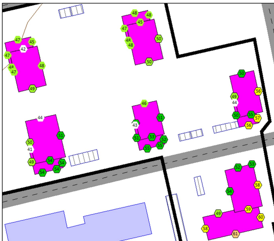
Kuva 17 Vaiheen 2. yöajan keskiäänitasot julkisivuilla.
