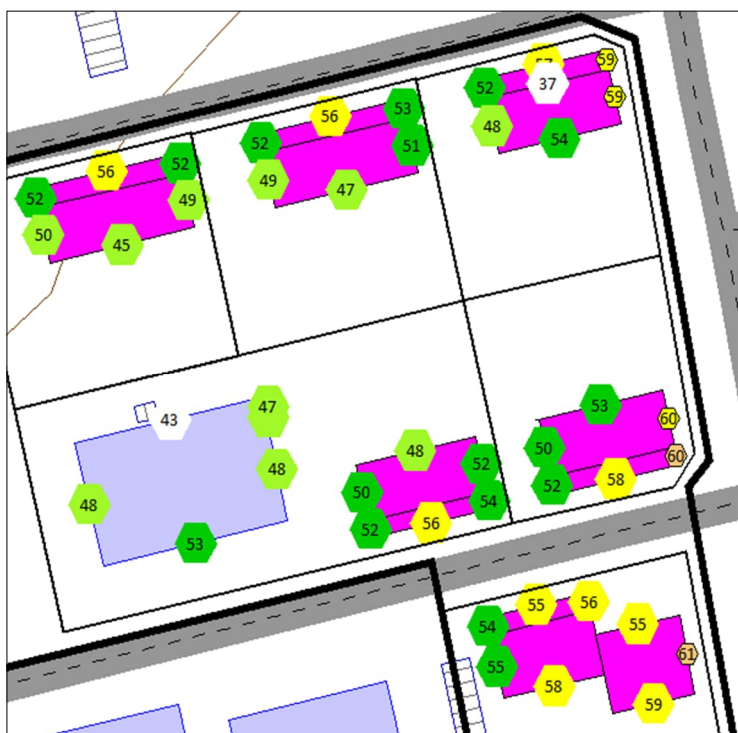
Kuva 7 Julkisivuille kohdistuvat korkeimmat keskiäänitasot ennustetilanteessa 2040 yöllä. Pistetaloversio.
