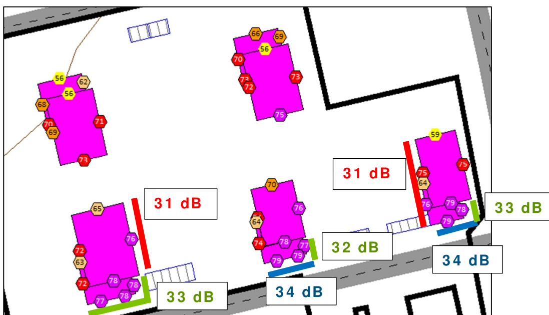
Kuva 21 Julkisivuille kohdistuvat ääneneristävyytsvaatimukset enimmäisäänitasojen LAF_{max} perusteella vaiheessa 1. niiltä osin, kun minimivaatimus 30 dB ylittyy.
