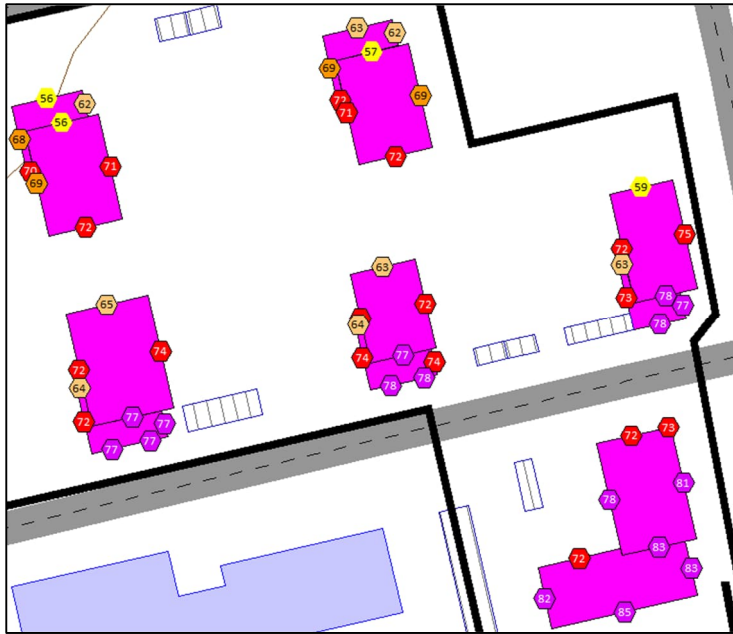
Kuva 19 Vaiheen 2. raideliikenteen aiheuttamat enimmäisäänitasot LAFmax julkisivuilla.
